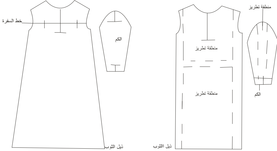
شكل (٢) رسم تخطيطي يوضح الخطوط الأساسية للجلباب
